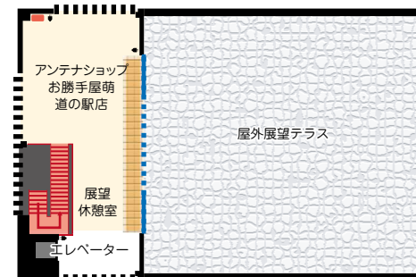
船場公園管理棟 2 F 平面図
